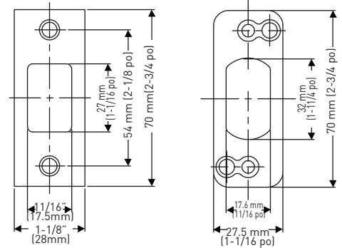
PLAQUE AVANT
