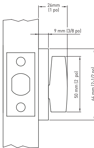
GARNITURE INTÉRIÈRE À PÊNE DORMANT
