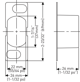
BOÎTE À POUSSIÈRE
