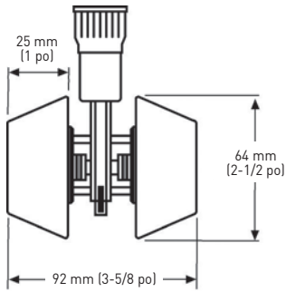
PÊNE DORMANT À DEUX BARILLETS
