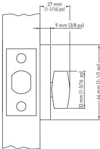
PÊNE DORMANT INTÉRIEUR MONOFAÇE
